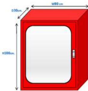
ตู้เก็บสายดับเพลิง Fire Hose Reel Fire Hose Rack
